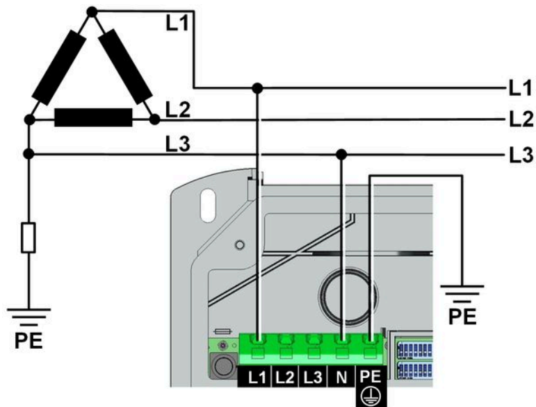
Raccordement à un système IT à trois conducteurs
